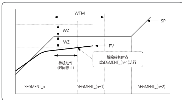
[图2] WAIT动作 - 在WTM以内解除待机动作的情况例
