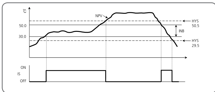
[图22] 内部信号动作例#1
