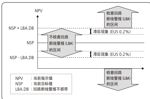
[图31] 回路断线警报不感带的动作
