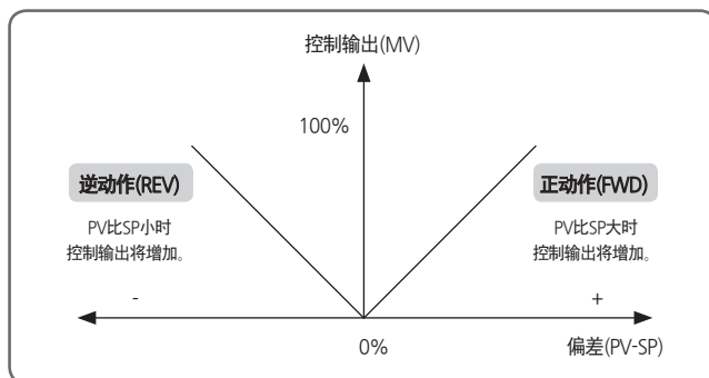
[图16] 正动作和逆动作
