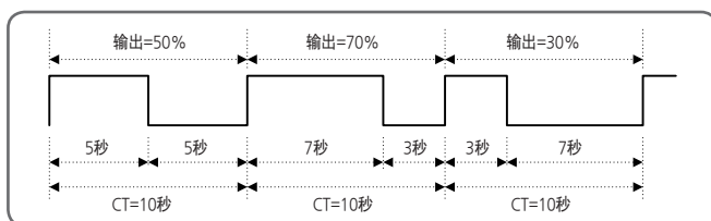
[图17] CT = 10秒时控制输出操作例
