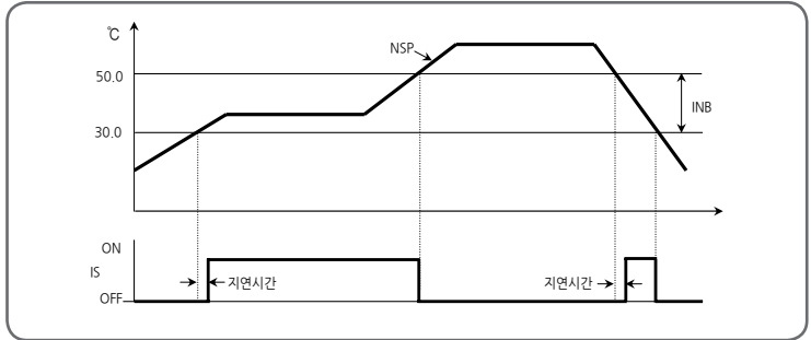
[图24] 内部信号动作例#3
