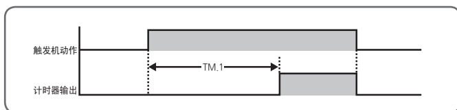
【图26】计时动作Delay 1
