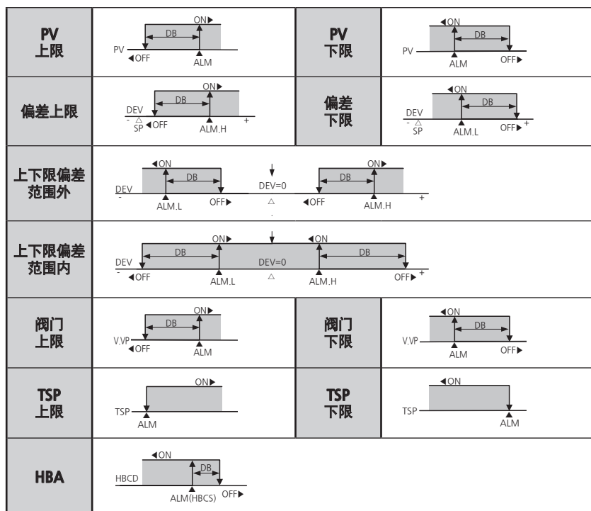
[图21] 警报操作
