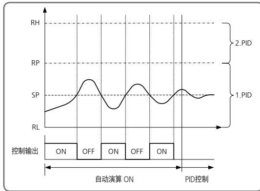
[图4] 自动演算
