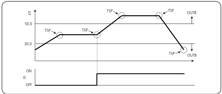
[图25] 内部信号动作例#4
