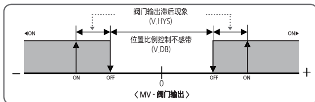
[图18] 位置比例控制阀门输出动作
