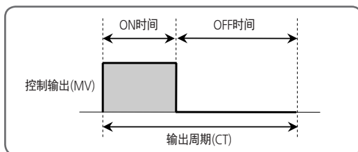
[图30] 取暖器断线警报检测条件
