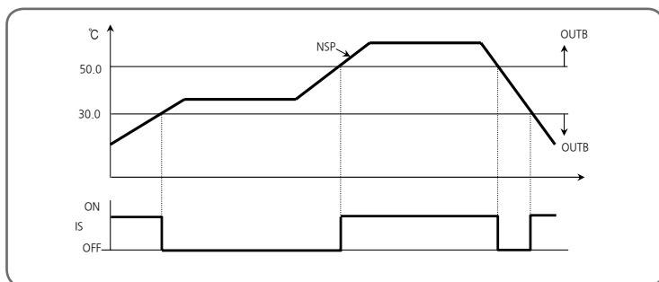
[图23] 内部信号动作例#2
