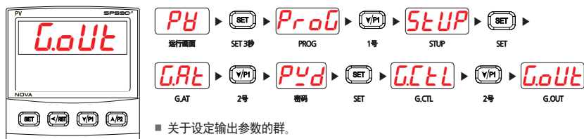
[表4] 输出种类
