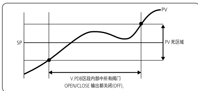
[图20] V.PDB(阀门PV死区域)
