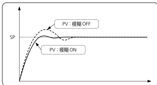
[图10] 由模糊功能抑制过冲
