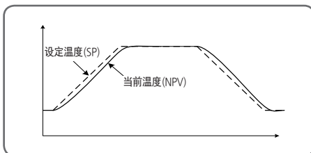
[图8] D.PV控制
