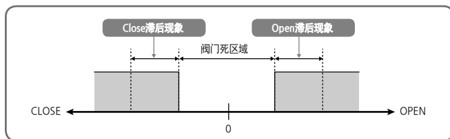
[图19] V.DB、V.HYS 操作
