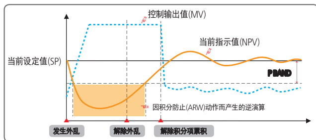
[图7] 有积分防止(ARW)功能的时候
