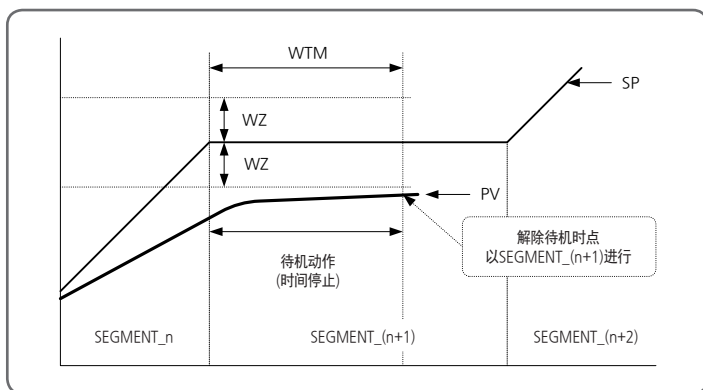
[图3] WAIT动作 - WTM 以内PV无法进入WZ的情况例
