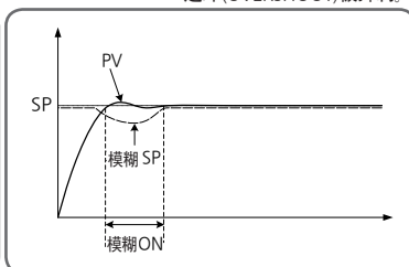
[图12] 模糊 ON
